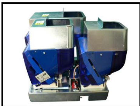
Cj. 3 descargadores (GTD) 21621430
